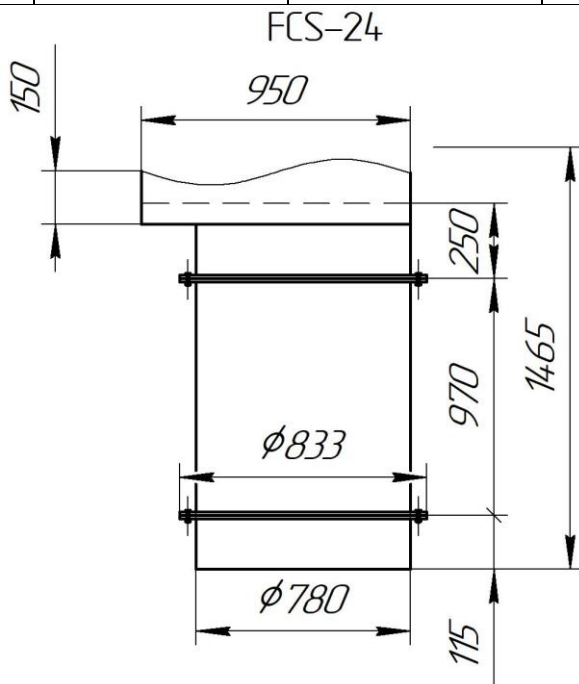
Рисунок 1 – Габариты фильтра FCS-24 (14)
